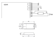
Technische Daten Philips HID-PV C 50 /I CDM 220-240V 50/60Hz für 50W
